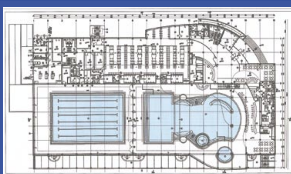
Tlocrt bazena: Prizemlje
